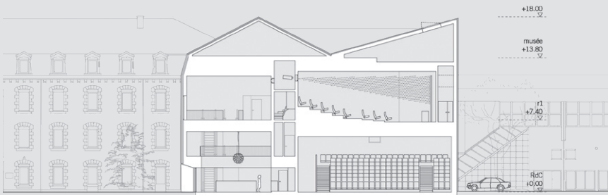
Snitt vest-øst
